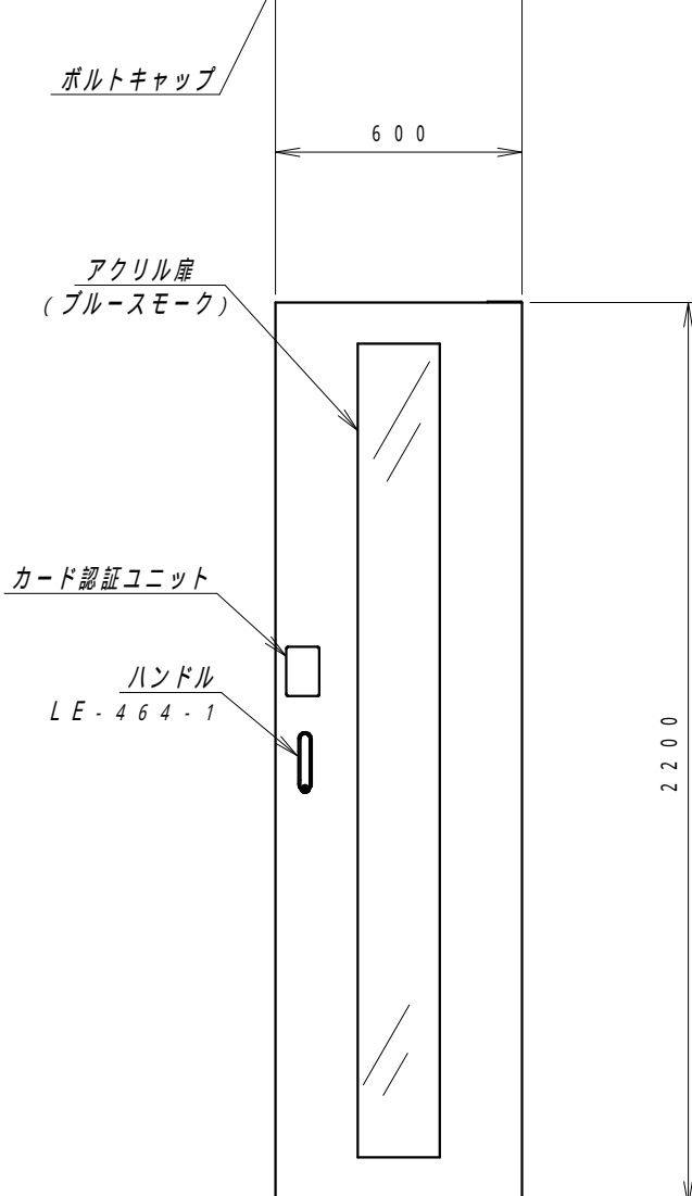
正面図 側面図 背面図 正面内観図
