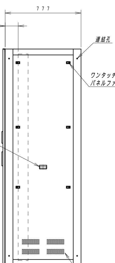
正面図 側面図 背面図 正面内観図
