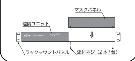
Lタイプ取付金具 FP-P101
