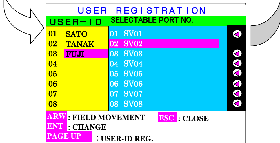
図-6 ユーザに対するサーバ使用許可設定画面
