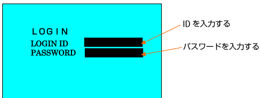
図-1 LOGIN 画面
