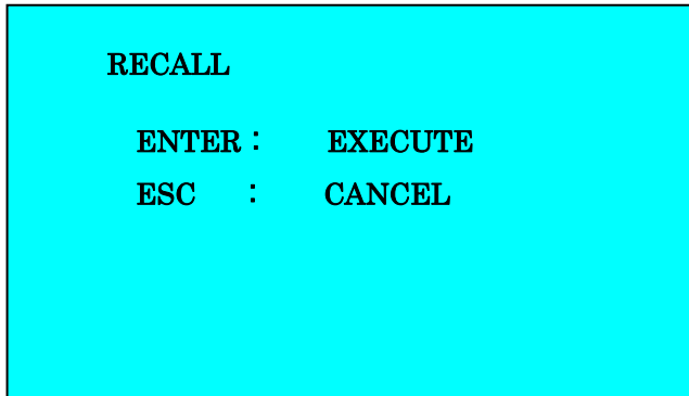
図-13 RECALL 画面
