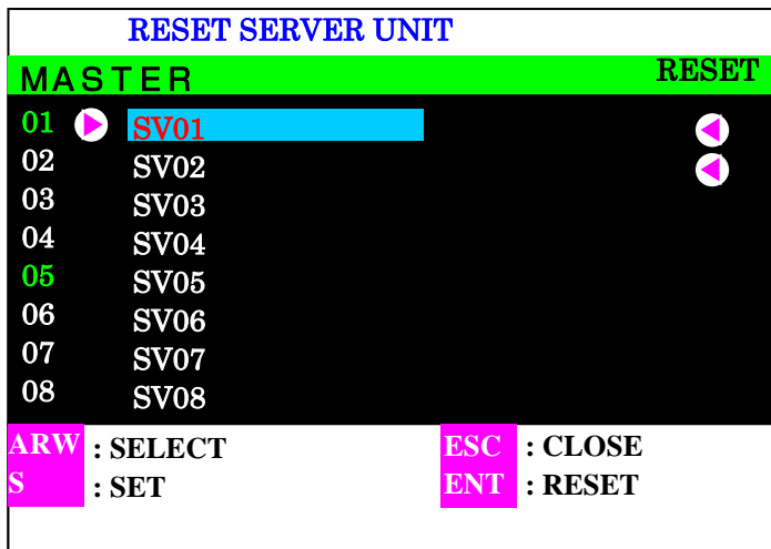
図-11 サーバユニットのリセット設定画面
