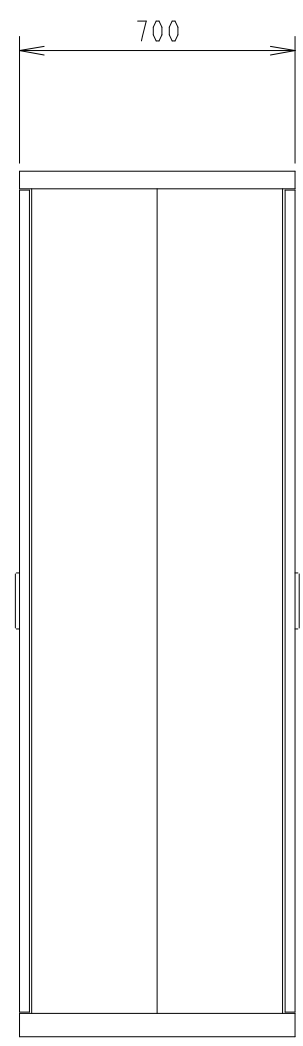
側面図
