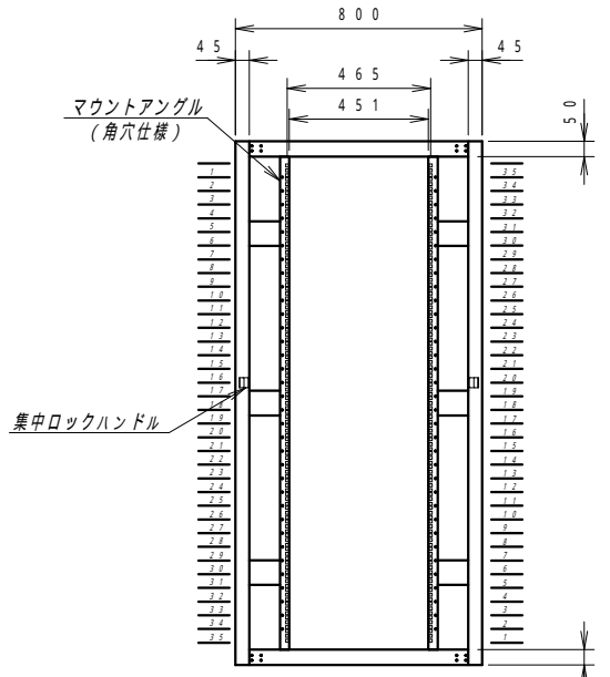
正面内観図
