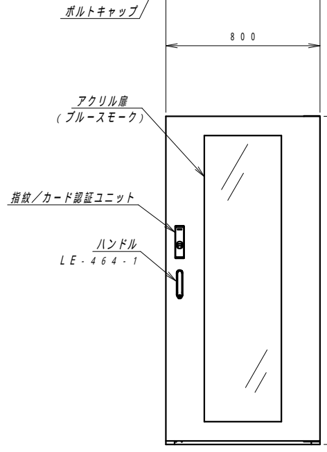
正面図
